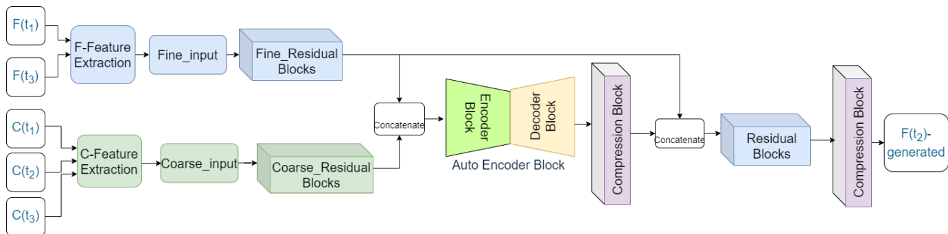
FIGURE 2 : Architecture du générateur S2S3-STFGAN.
