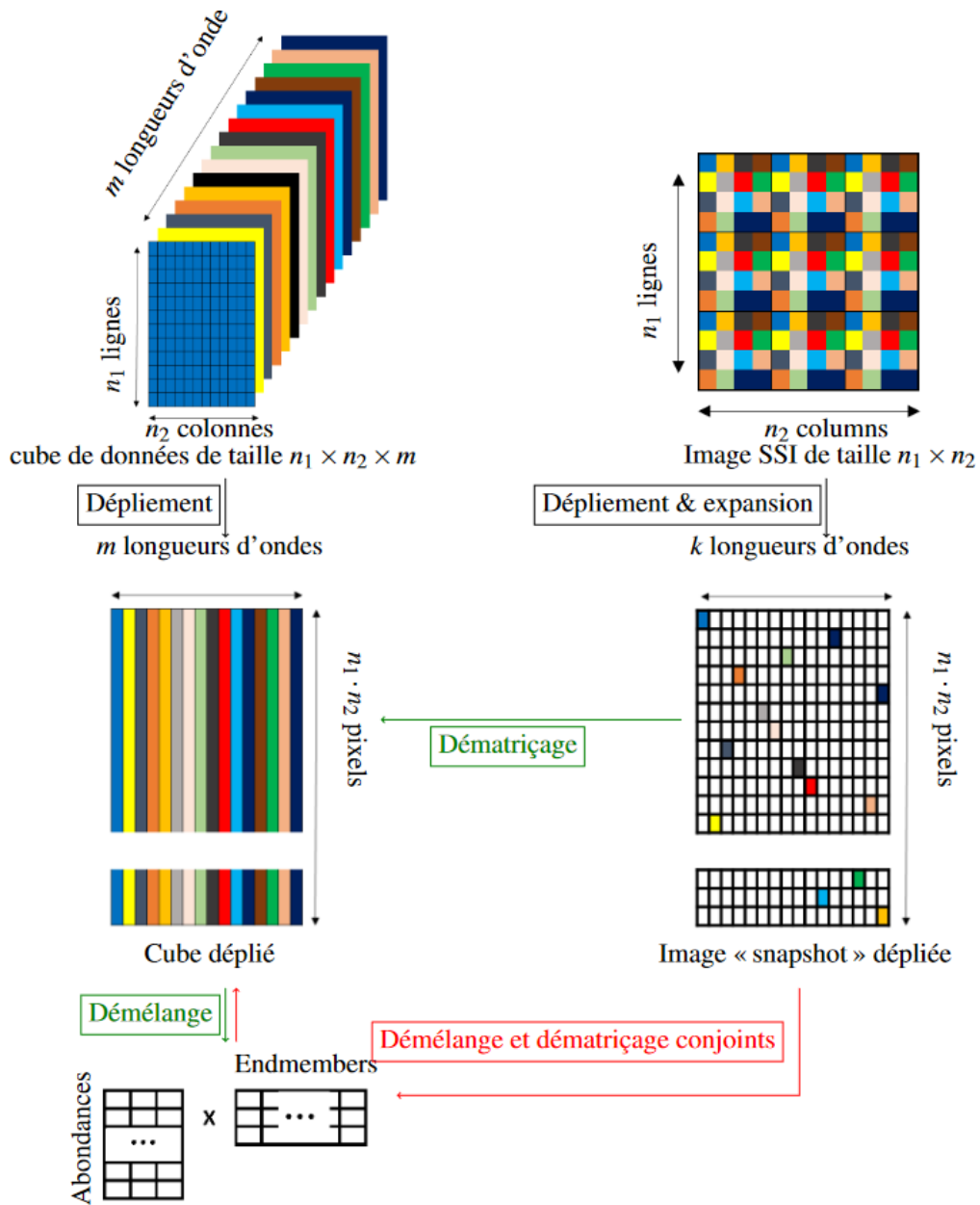
FIGURE 6.13 – Principes du démixage post-dématricage (en vert) et du dématricage et démixage conjoints (en rouge).
